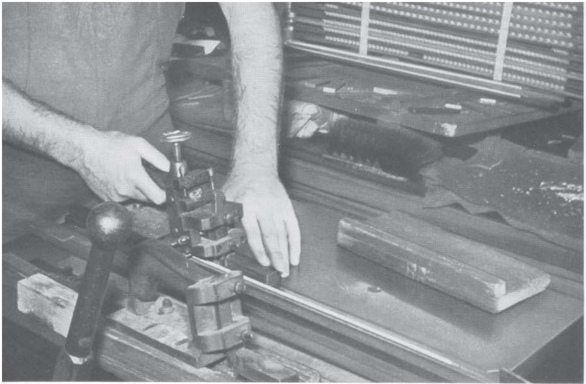
Der Fertigmacher beim Bestoßen der Schrift
