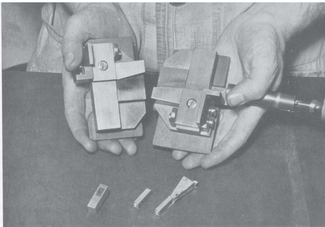
Das Handgießinstrument, davor links die Mater, rechts ein Buchstabe mit Anguß
